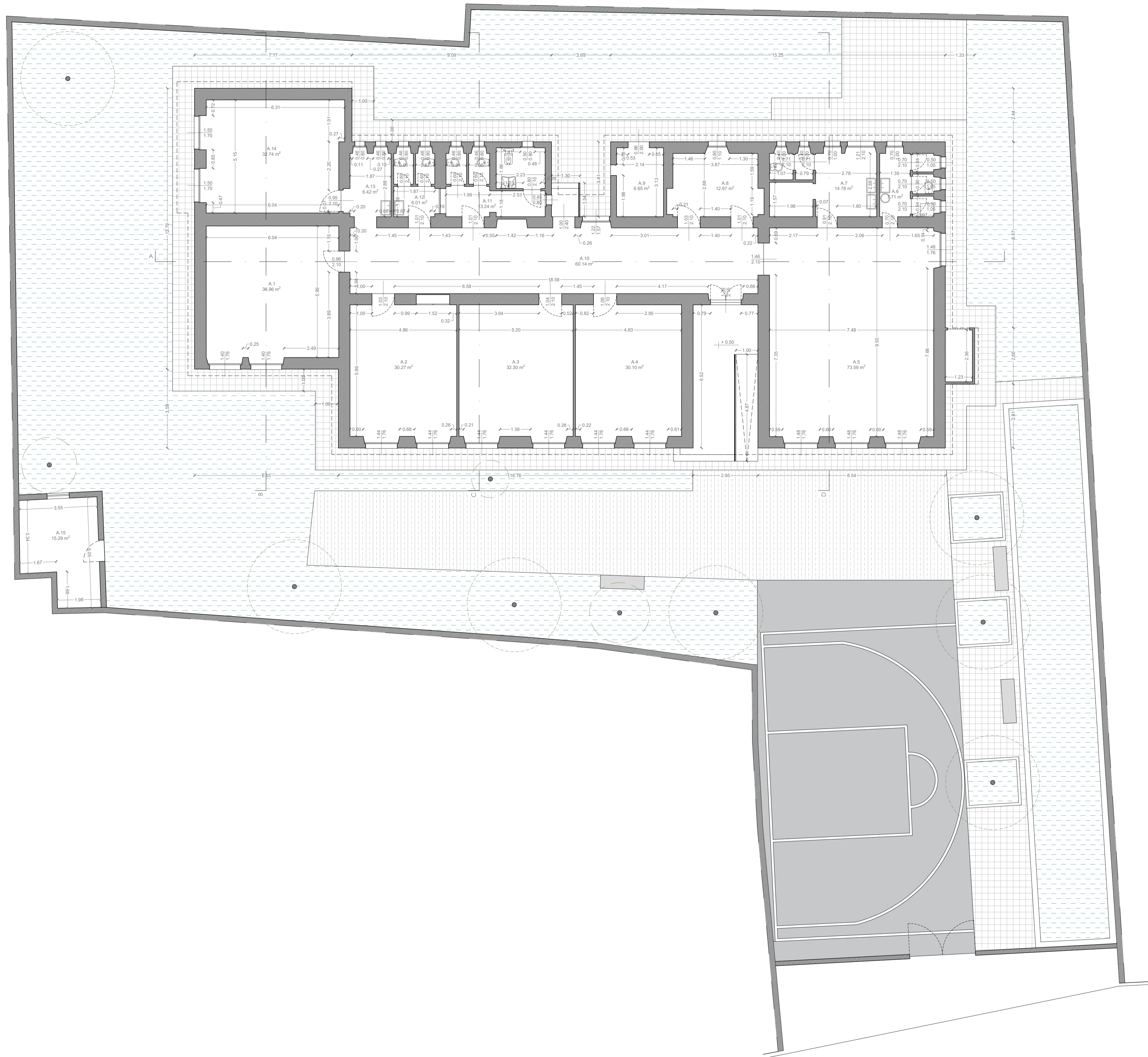
PIANTA PIANO TERRA STATO DI FATTO
