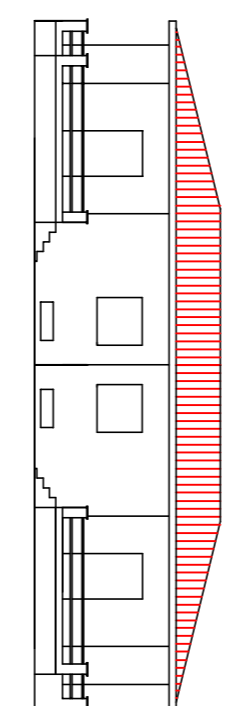
TIPOLOGIA SINGOLA B1 (1P) PROSPETTO POSTERIORE
