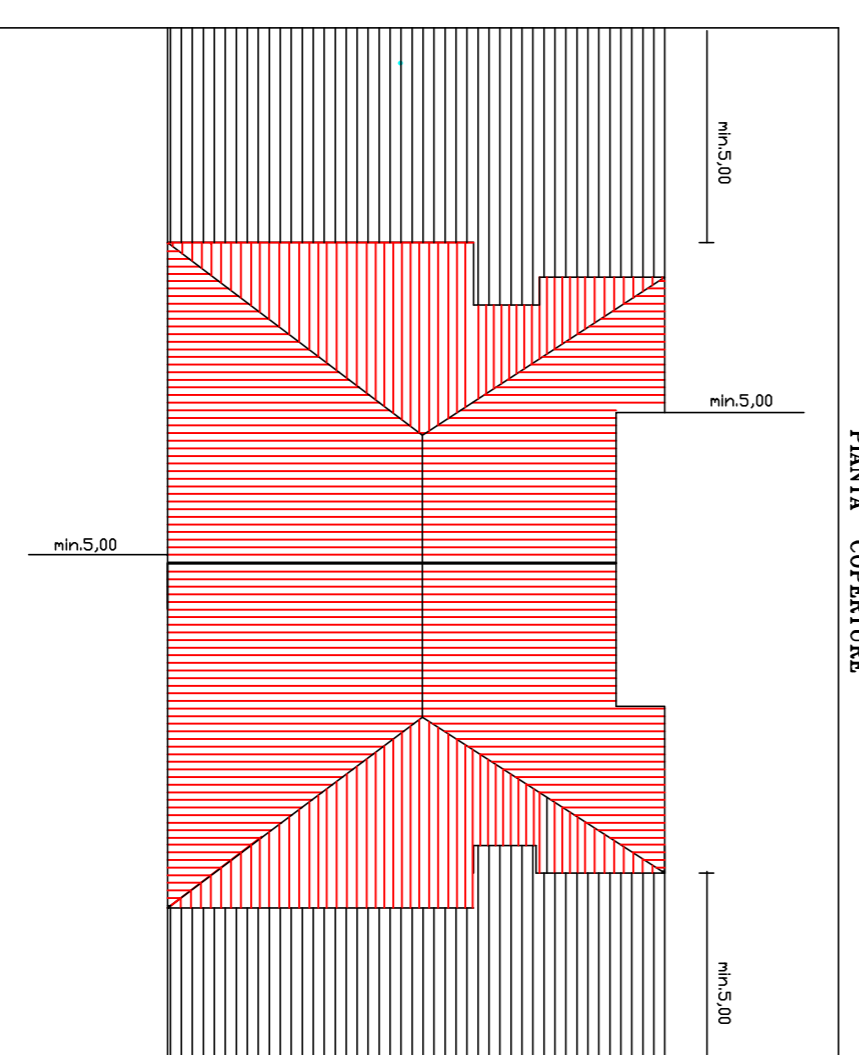
TIPOLOGIA SINGOLA-BINATA B2 PIANTA COPERTURE
