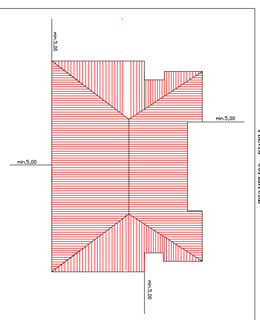
TIPOLOGIA SINGOLA-BINATA B1 PIANTA COPERTURE
