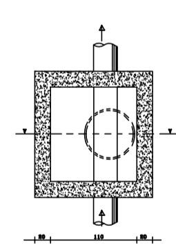
PART. POZZETTO ISPEZIONE FOGNE PLUVIALI
