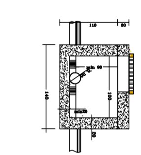
PART. POZZETTO INCROCIO FOGNE NERE
