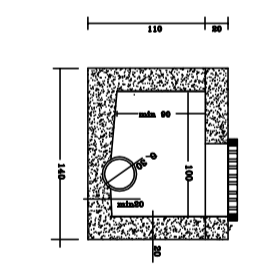
PART. POZZETTO ISPEZIONE FOGNE PLUVIALI
