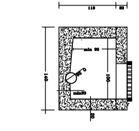
PART. POZZETTO ISPEZIONE FOGNE NERE
